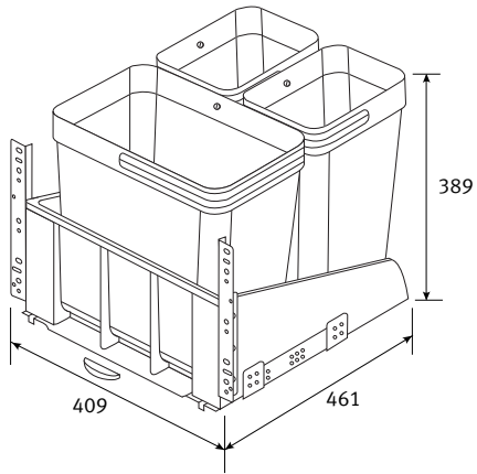
Sorter 700 K 45/M 45
