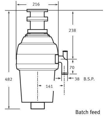
Franke Turbo WD-1001B 134.0049.851
