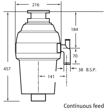
Franke Turbo WD-1001 134.0049.850
