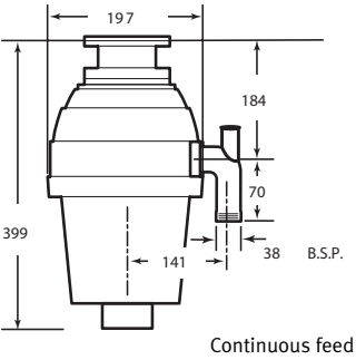
Franke Turbo WD-500 134.0049.848
