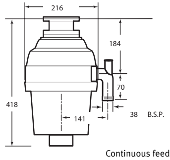
Franke Turbo WD-751 134.0049.849
